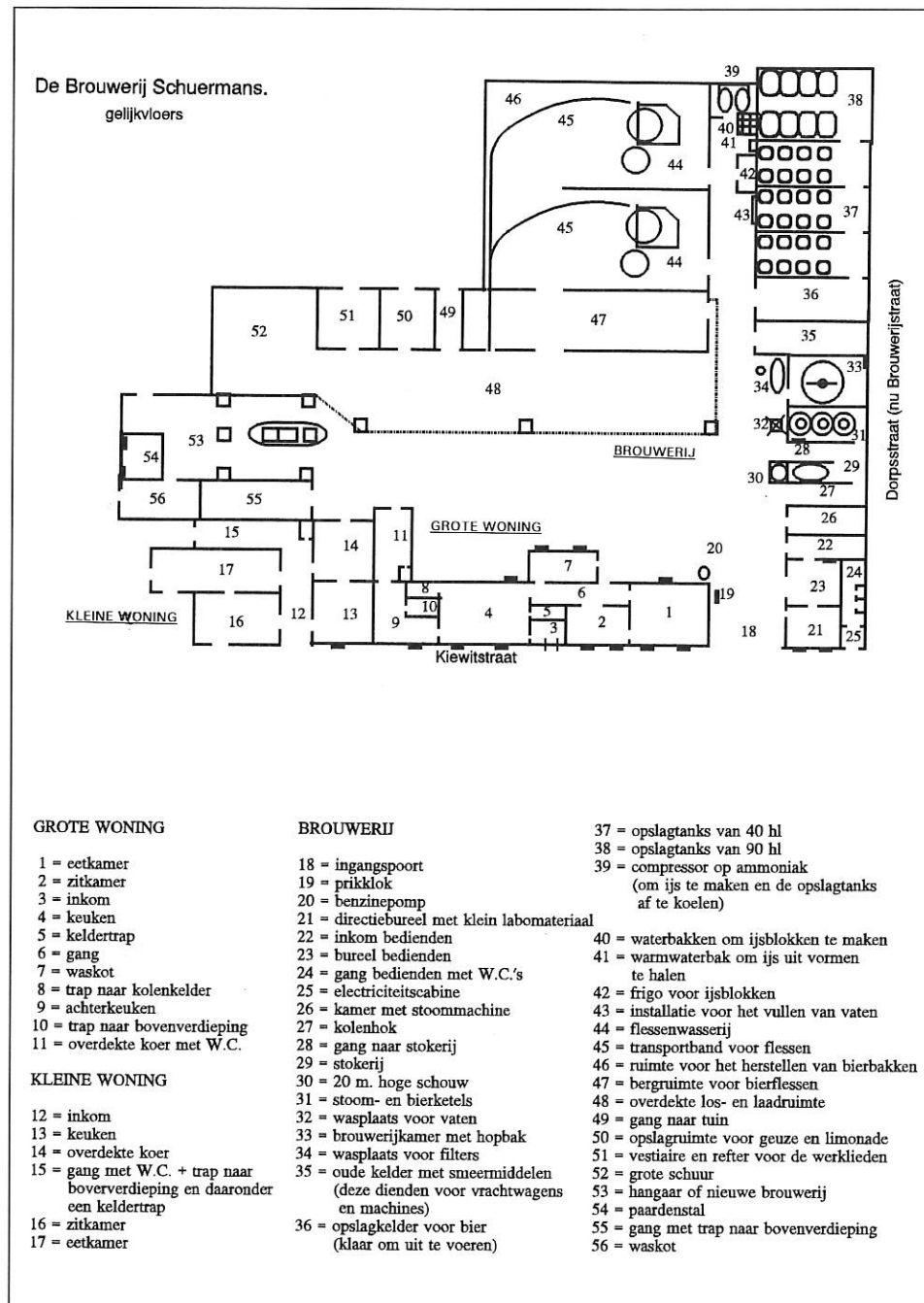
4. Plattegrond van de industriële brouwerij N.V. Schuermans te Kortenbergh (Collectie Cultuur-Historische Vereniging van Erps-Kwerps)
